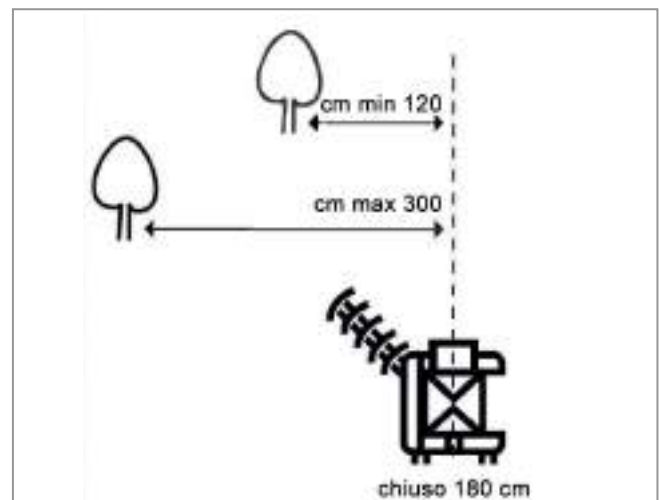
LARGHEZZA DI LAVORO FRUTTETO VERSIONE 2
